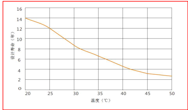
不同温度下的浮充设计寿命曲线
