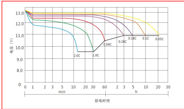
不同倍率下的放电曲线
