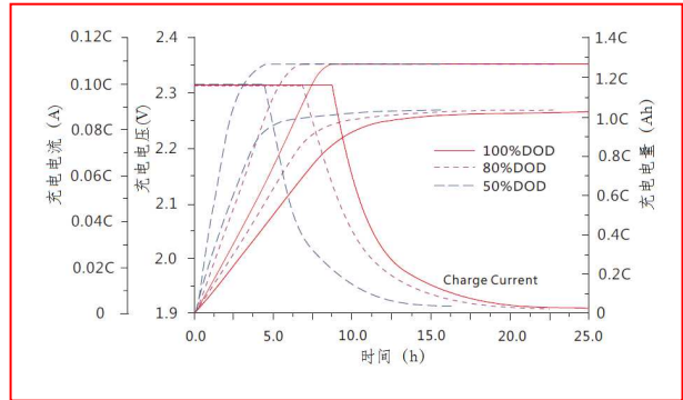
不同放电深度下的充电曲线
