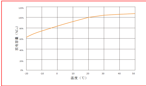
不同温度下的放电容量曲线
